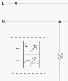
Для ламп накаливания, галогенных и регулируемых компактных ламп (220 В)
