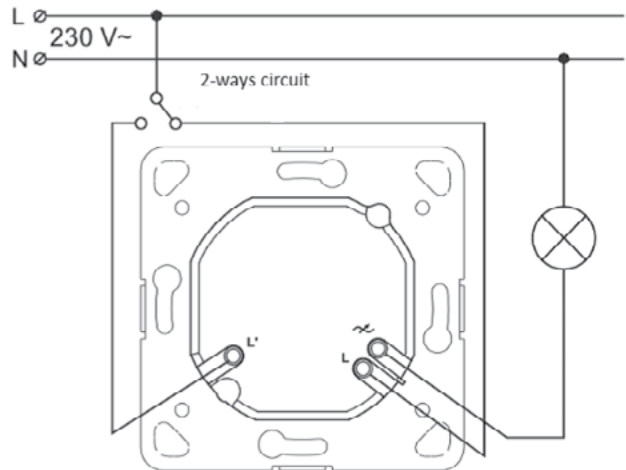
Переключение на два направления
