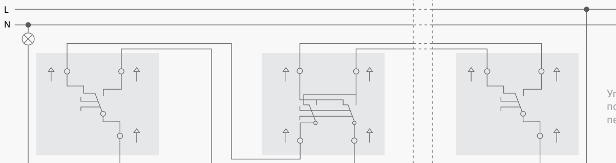
ПЕРЕКЛЮЧАТЕЛЬ 1-КЛАВИШНЫЙ
