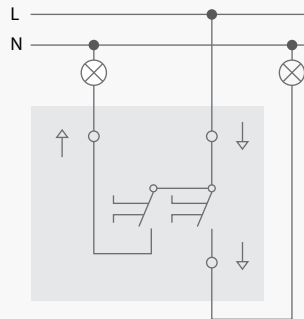
ВЫКЛЮЧАТЕЛЬ 2-КЛАВИШНЫЙ
