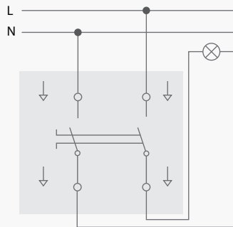
ВЫКЛЮЧАТЕЛЬ 1-КЛАВИШНЫЙ, 2-ПОЛЮСНЫЙ
