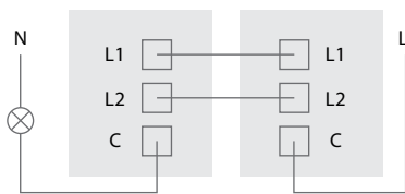
СВЕТОРЕГУЛЯТОР ПЕРЕКЛЮЧАТЕЛЬ
