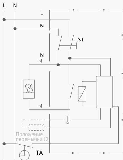
КОМНАТНЫЙ ТЕРМОСТАТ
