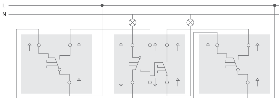
ПЕРЕКЛЮЧАТЕЛЬ 1-КЛАВИШНЫЙ
