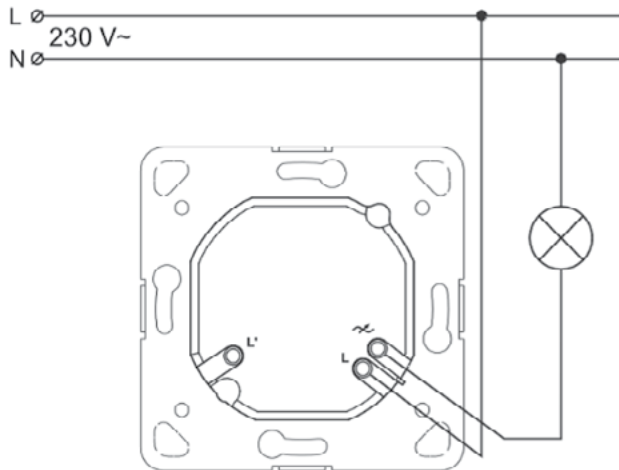
Типичное подключение к сети
