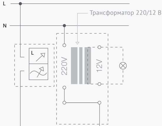
Для галогенных ламп (12 В), подключенных через трансформатор
