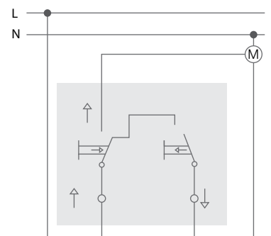
ВЫКЛЮЧАТЕЛЬ ДЛЯ ЖАЛЮЗИ 2-КЛАВИШНЫЙ
