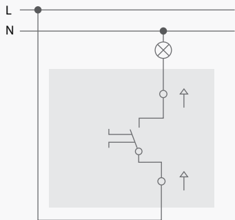
ВЫКЛЮЧАТЕЛЬ 1-КЛАВИШНЫЙ
