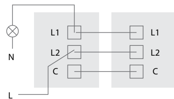
СВЕТОРЕГУЛЯТОР ПЕРЕКЛЮЧАТЕЛЬ
