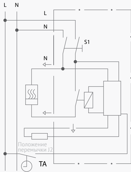
ТЕРМОСТАТ ДЛЯ ПОЛА
