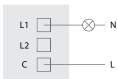
Цепь одностороннего подключения
