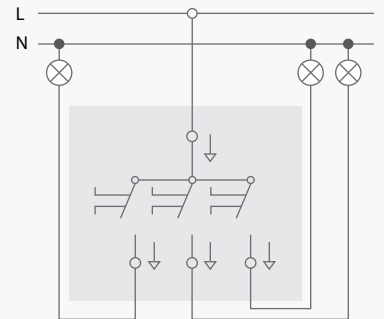
ВЫКЛЮЧАТЕЛЬ 3-КЛАВИШНЫЙ
